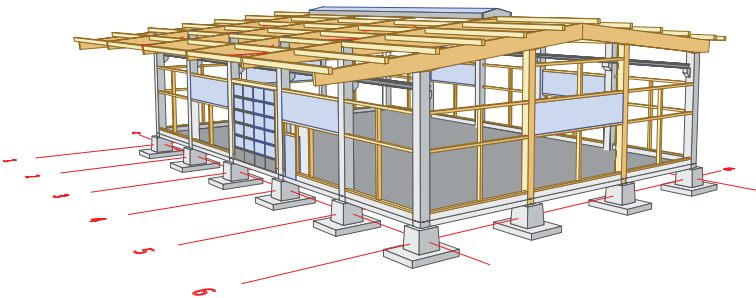
Konstruktiver Aufbau der BSflexiHalle in der Basisversion
